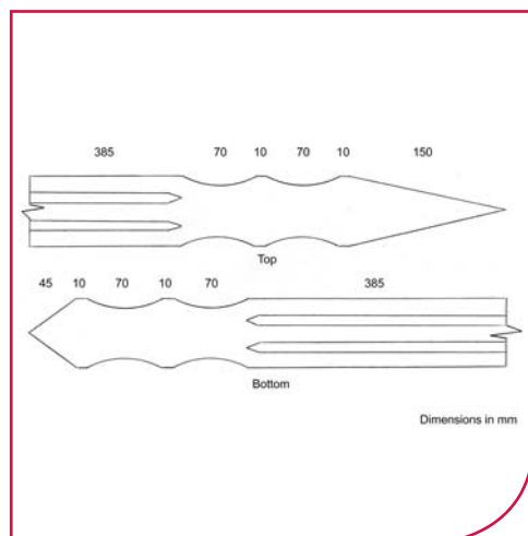
6. FIN 2 and FIN 3 product dimensions
