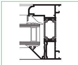
Fixed light jamb
