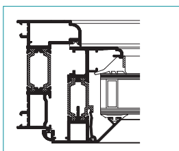
Jamb/vent
